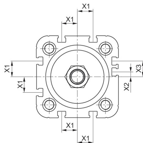
CCI-PC ø50-ø63
