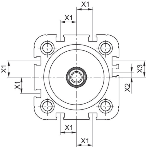
CCI-PC ø50-ø63
