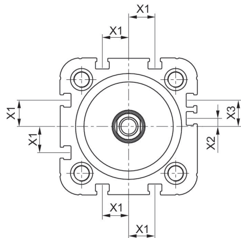
CCI-PC ø50-ø63
