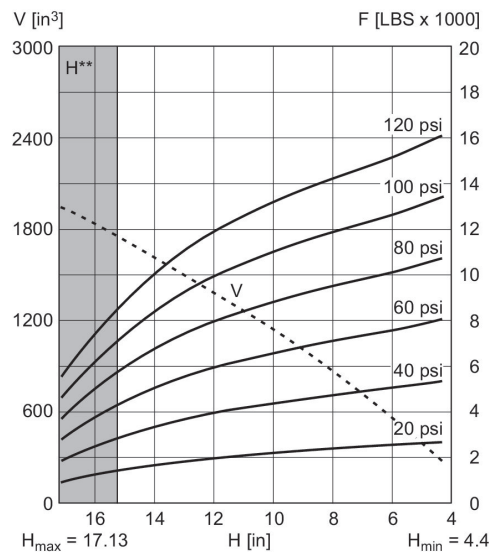
Diagrama força-percurso R432039296
