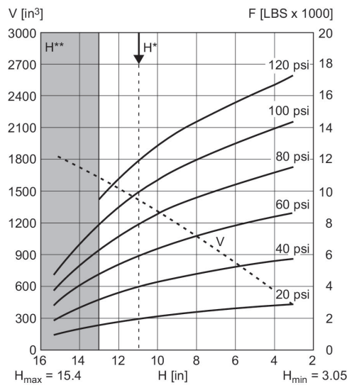
Diagrama força-percurso R432039770
