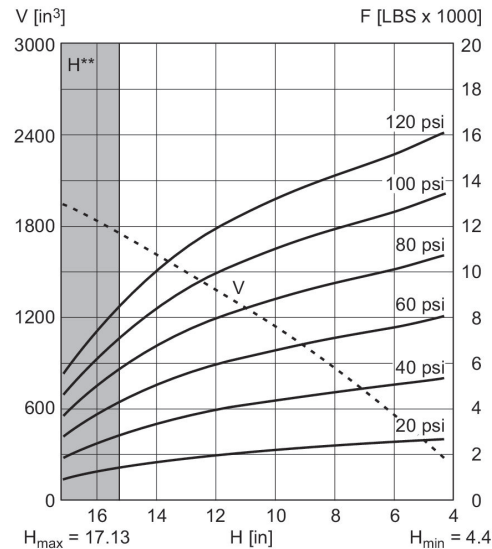
Diagramma forza-corsa R432039296
