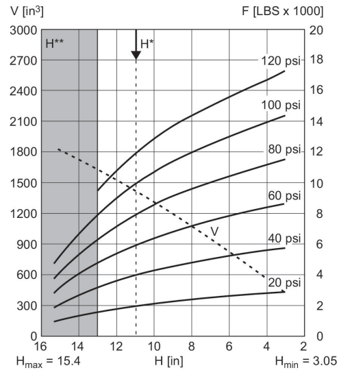
Diagramma forza-corsa R432039770
