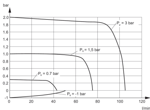
Diagramme du débit pour plage de pression jusqu'à 2 bar
