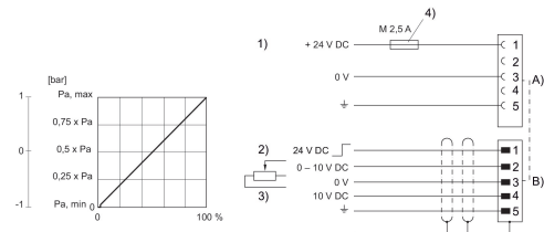
Fig. 3 Kennlinie und Steckerbelegung für Potentiometer-Ansteuerung ohne Istwertausgang
