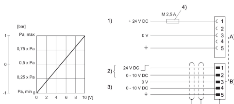
Fig. 2 実際値出力付電圧制御の特性とプラグ割り当て
