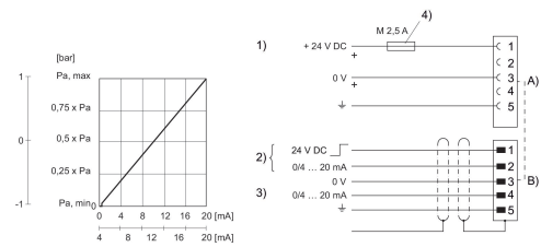
Fig. 1 実際値出力付電流制御の特性とプラグ配置
