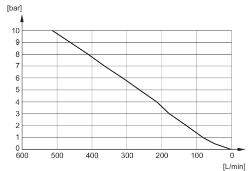
Diagrama de caudal 1827430004
