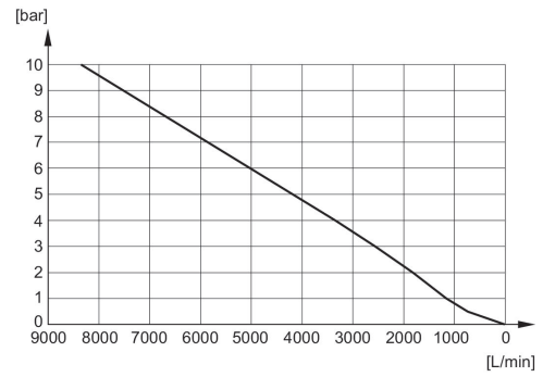
Diagrama de caudal R412007878
