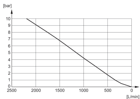
Diagrama de fluxo R412007876
