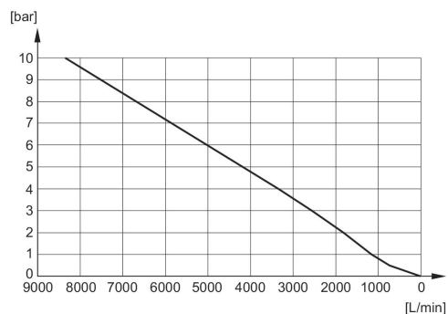
Diagrama de fluxo R412007878
