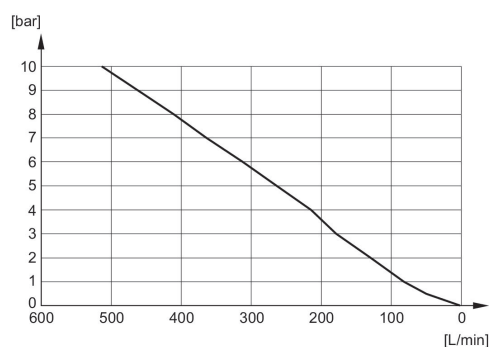
Diagrama de fluxo 1827430004
