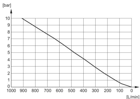
Diagrama de fluxo R414000155
