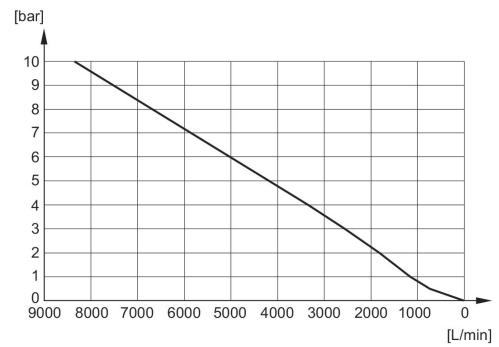
Diagramma della portata R412007878
