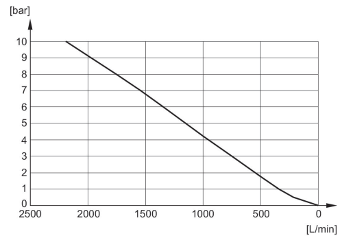
Diagramma della portata R412007876
