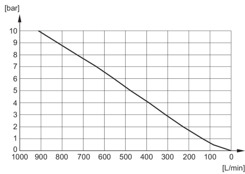
Diagramma della portata R414000155
