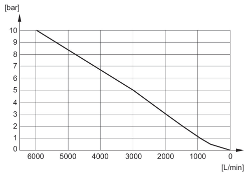
Diagramma della portata R412007877
