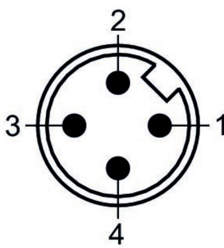
Polbild Stecker
