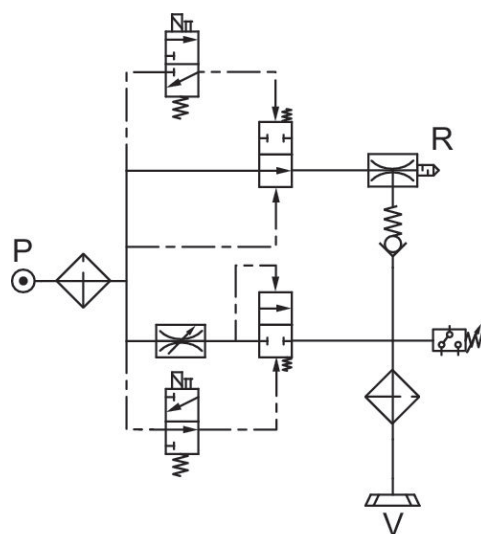
esquema de conexiones ECD-LV-...NO
