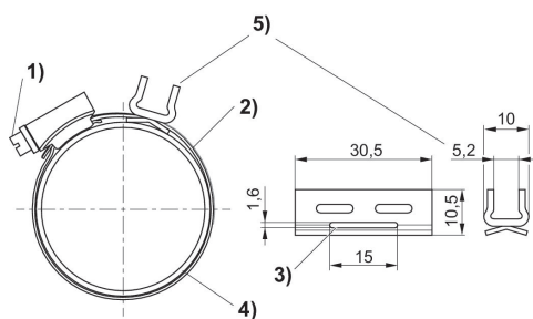
1) Befestigungsschraube 2) Spannband 3) Durchlass für Spannband 4) Zylinderrohr 5) Sensorhalterung
