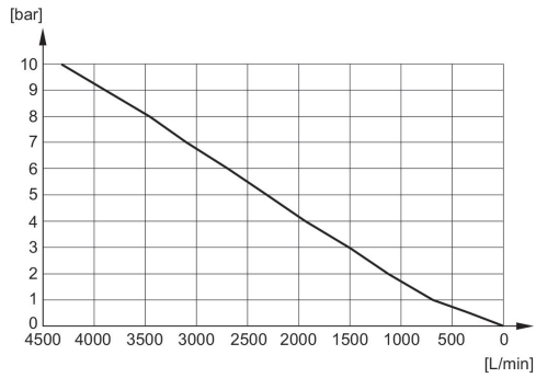
Durchflussdiagramm R412010245
