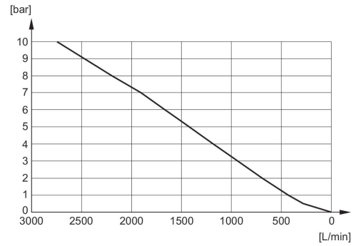
Durchflussdiagramm R412010283
