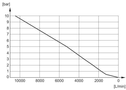
Durchflussdiagramm R412010247
