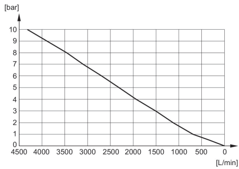
Durchflussdiagramm R412010245
