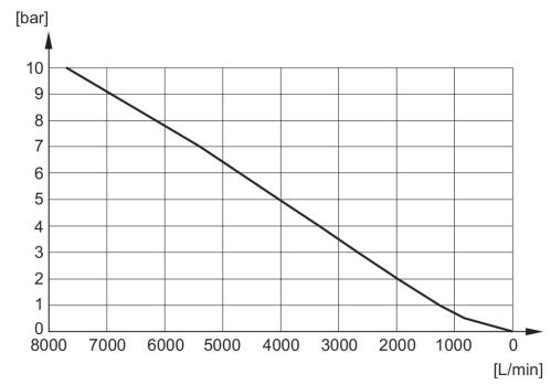
Durchflussdiagramm R412010246
