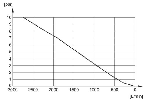
Durchflussdiagramm R412010283
