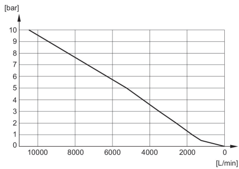
Diagramme du débit R412010247
