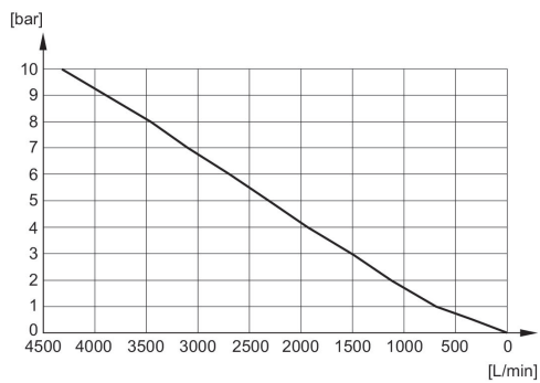
Diagramme du débit R412010245
