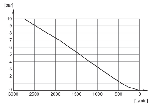
Diagramme du débit R412010283
