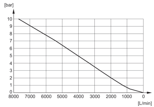
Diagramme du débit R412010246
