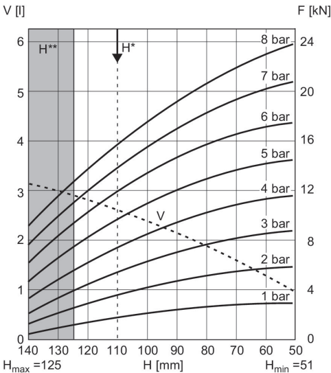
Diagrama força-percurso R412010218
