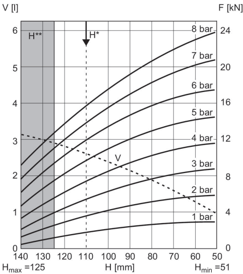
Diagramma forza-corsa R412010218
