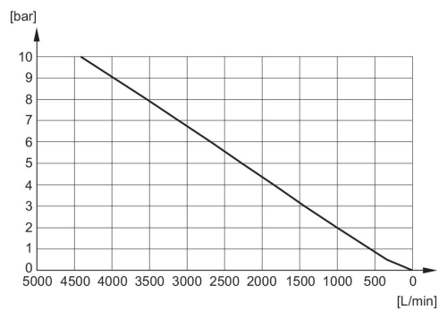
Diagramma della portata R412010083
