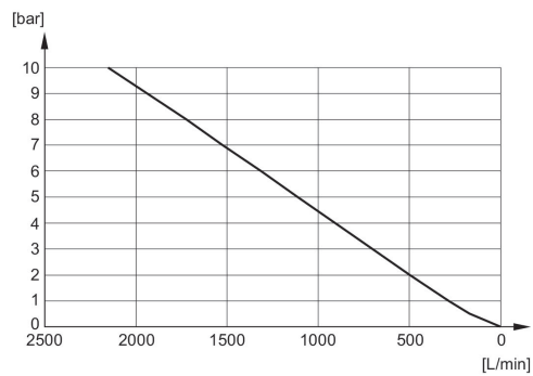
Diagramma della portata R412010081
