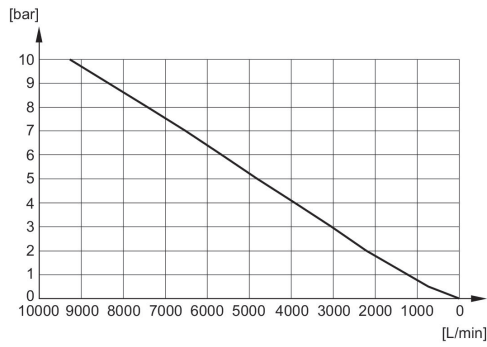
Diagrama de caudal R412010084
