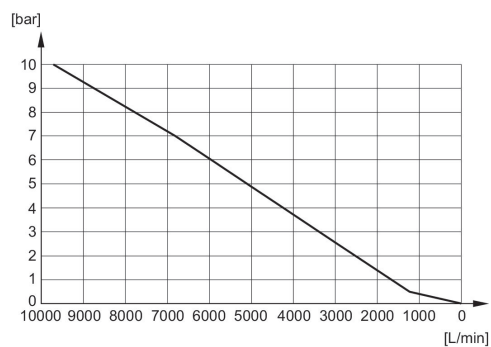
Diagrama de caudal R412010085
