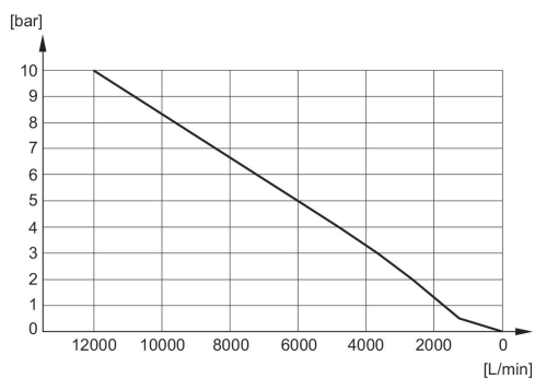
Diagrama de caudal R412010086
