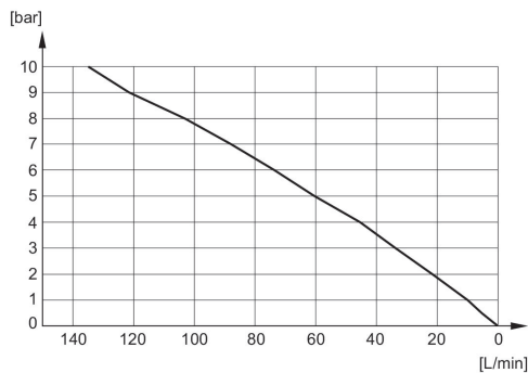
Diagrama de caudal R412010090
