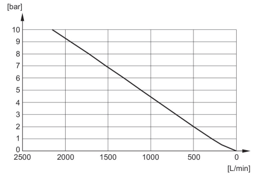
Diagrama de caudal R412010081
