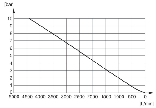
Diagrama de caudal R412010083
