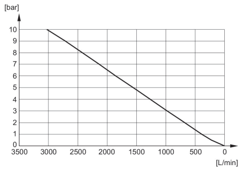
Diagramma della portata R412010082
