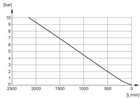
Diagrama de fluxo R412010081
