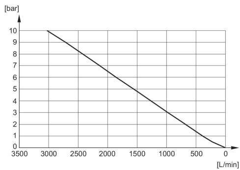
Diagrama de fluxo R412010082
