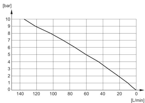
Diagrama de fluxo R412010090
