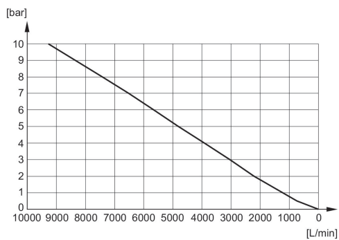
Diagrama de fluxo R412010084
