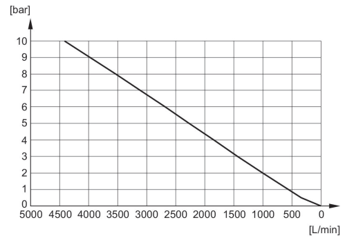
Diagramma della portata R412010083
