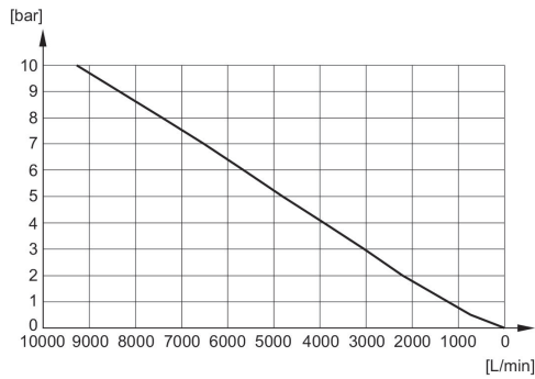
Diagramma della portata R412010084
