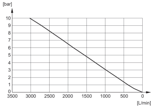
Diagramma della portata R412010082
