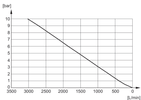
Diagramme du débit R412010082
