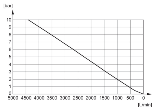
Diagramme du débit R412010083
