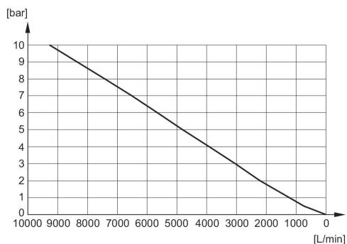
Diagramme du débit R412010084
