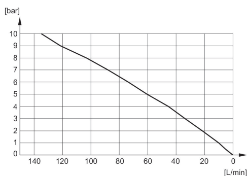
Diagramme du débit R412010090
