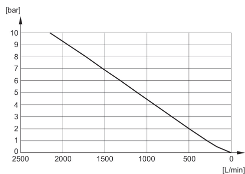
Diagramme du débit R412010081
