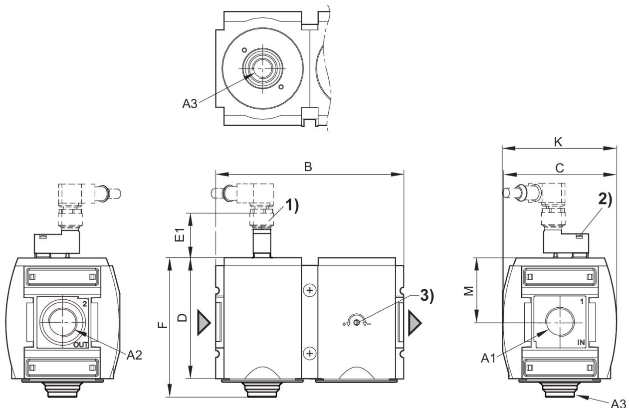
Fig. 4: Befüllleinheit mit Vorsteuerventil, Steckanschluss M12x1
