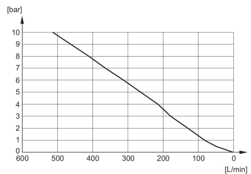
Diagrama de fluxo 1827430004
