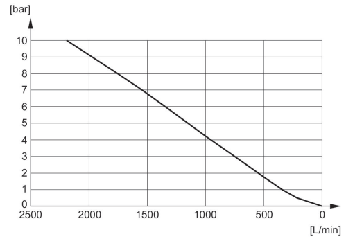
Diagrama de fluxo R412007876
