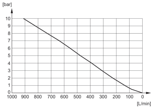
Diagrama de fluxo R414000155
