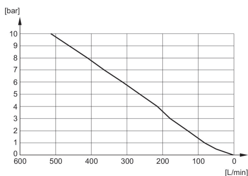
Diagramma della portata 1827430004
