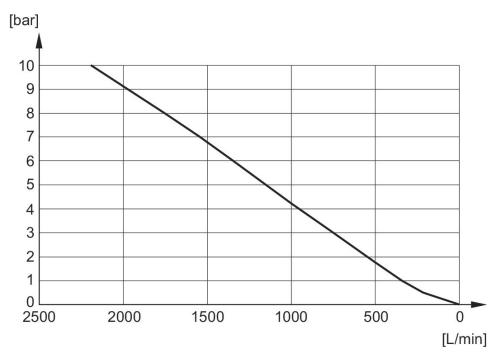
Diagramma della portata R412007876
