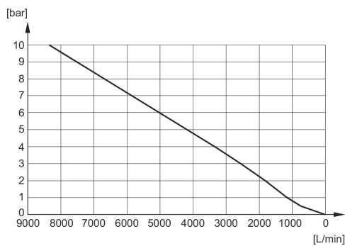
Diagramme du débit R412007878
