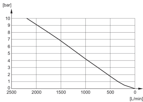
Diagramme du débit R412007876
