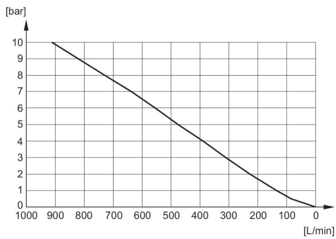
Durchflussdiagramm R414000155
