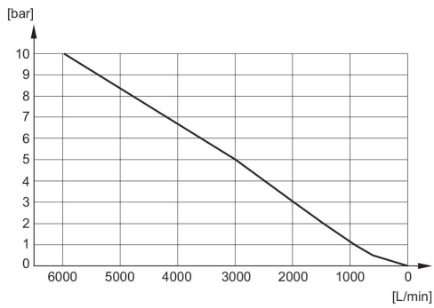
Durchflussdiagramm R412007877
