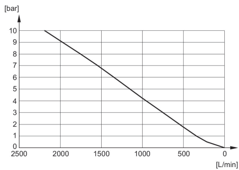
Diagrama de caudal R412007876
