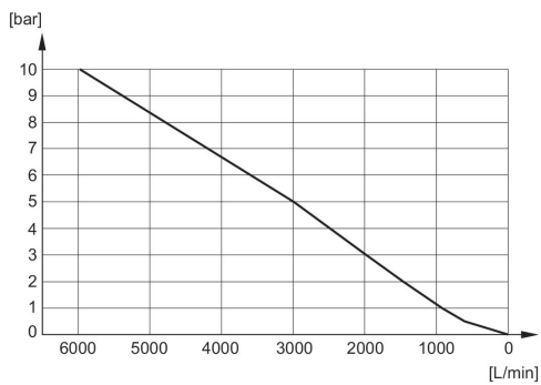
Diagrama de caudal R412007877
