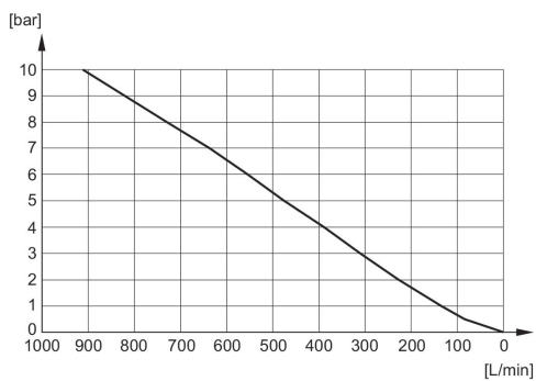
Diagrama de caudal R414000155
