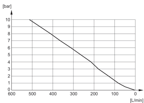
Diagrama de caudal 1827430004
