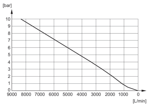
Diagrama de caudal R412007878
