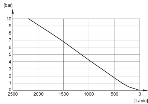
Diagramme du débit R412007876
