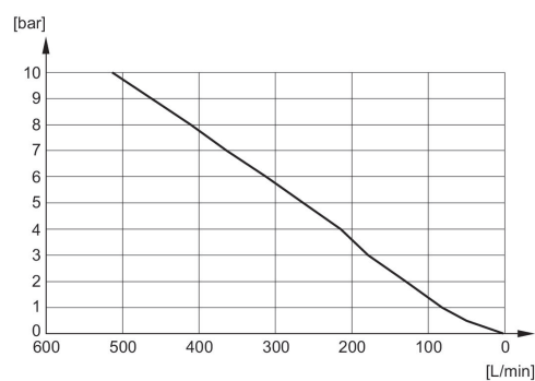
Diagramme du débit 1827430004
