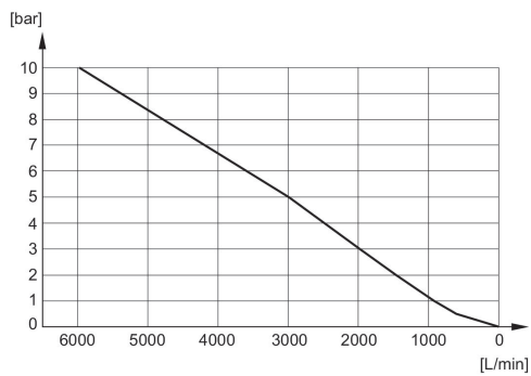
Diagramme du débit R412007877
