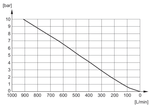
Diagramme du débit R414000155
