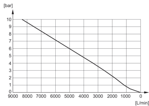
Diagramme du débit R412007878
