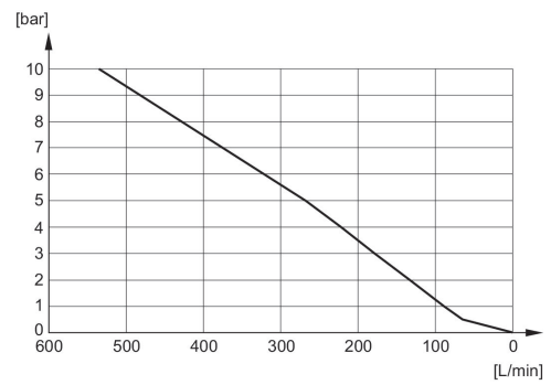
Diagrama de caudal R412007519
