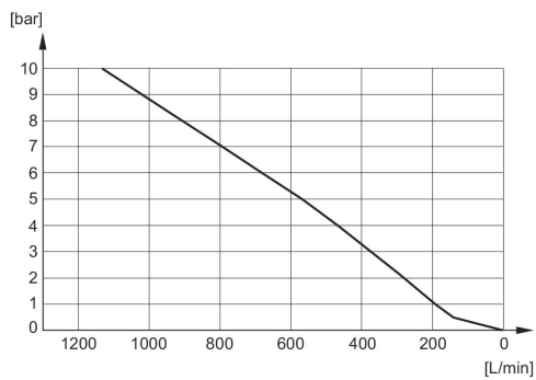
Diagrama de fluxo R412007899
