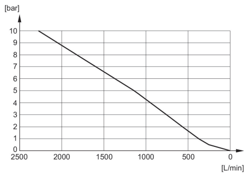
Diagrama de fluxo R412007520
