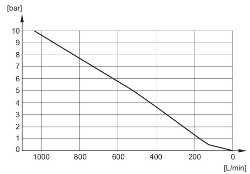
Diagrama de fluxo R412000591
