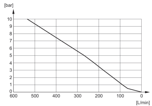
Diagrama de fluxo R412007519
