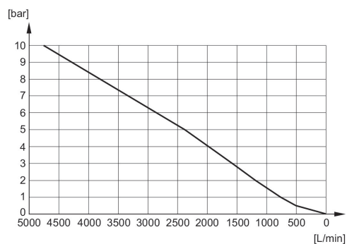
Diagramma della portata R412000593
