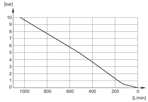
Diagramma della portata R412000591
