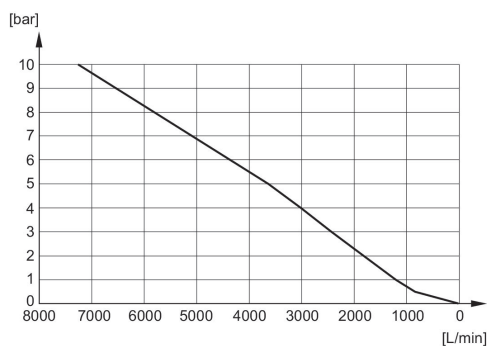
Diagramma della portata R412007715
