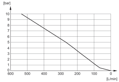
Diagramma della portata R412007519
