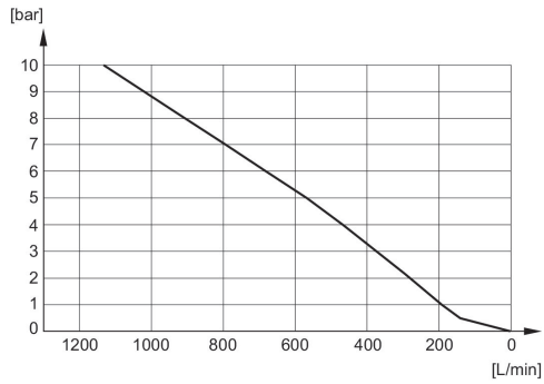
Diagramma della portata R412007899
