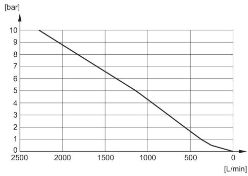
Diagramma della portata R412007520
