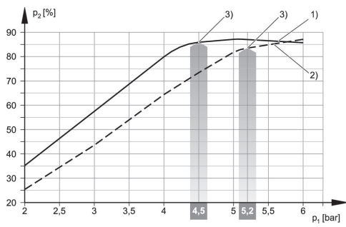
1) = Ø Düse 2,0 mm 2) = Ø Düse 2,5 mm 3) optimaler Betriebsdruck
