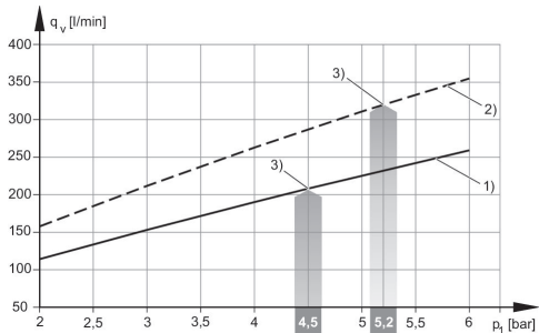
1) = Ø bocal 2,0 mm 2) = Ø bocal 2,5 mm 3) pressão de serviço ideal
