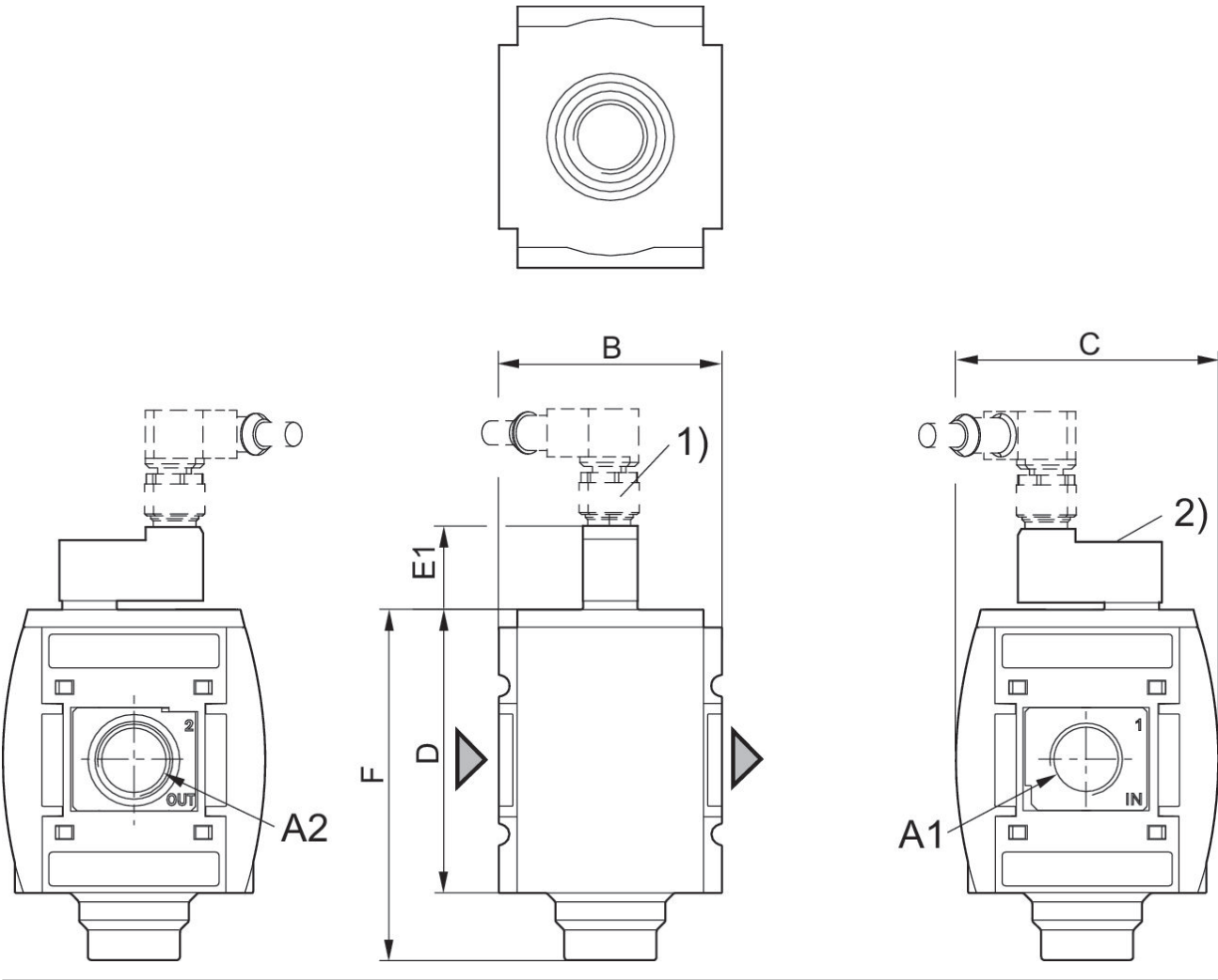
Fig. 2: válvula distribuidora 2/2 con válvula de pilotaje previo, conexión por enchufe M12x1
