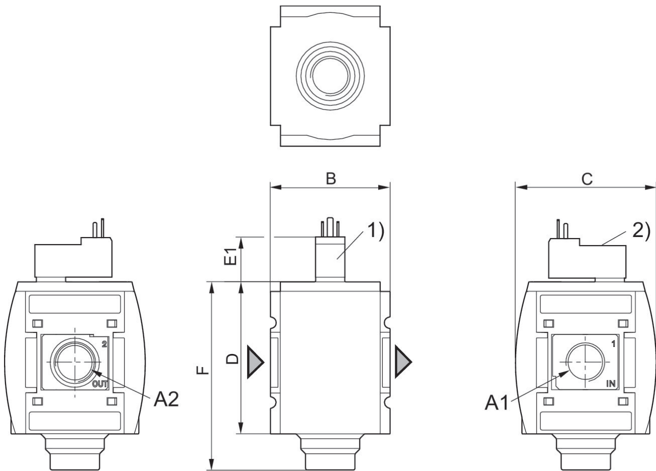
Fig. 1 : distributeur 2/2 avec distributeur pilote et orifice pour connecteur forme C
