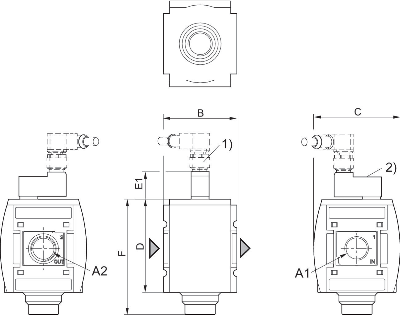
Fig. 2 : distributeur 2/2 avec distributeur pilote, raccord instantané M12x1
