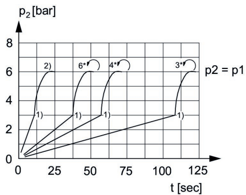
Andamento pressione secondaria durante il caricamento
