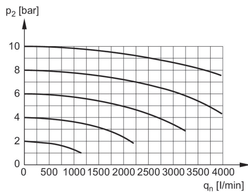
Caratteristica della portata
