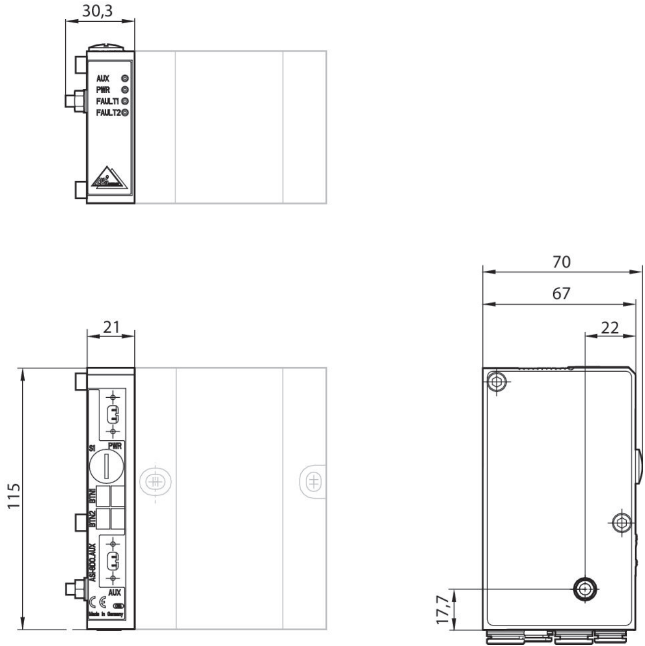
AS-i, 8DO-AUX
