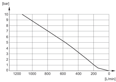
Diagrama de caudal R412007899
