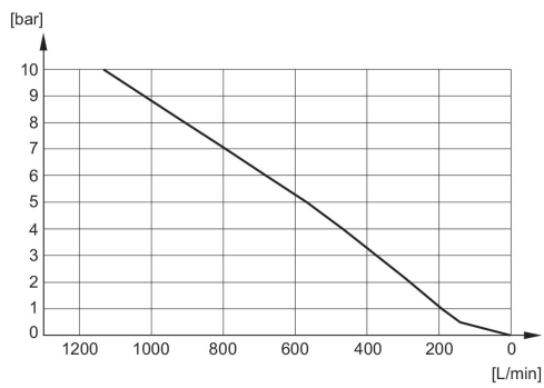
Diagramme du débit R412007899
