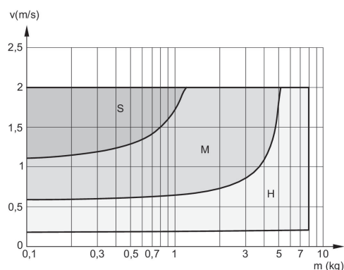
阻尼图 Ø 16 mm
