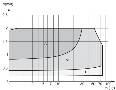
阻尼图 Ø 50 mm
