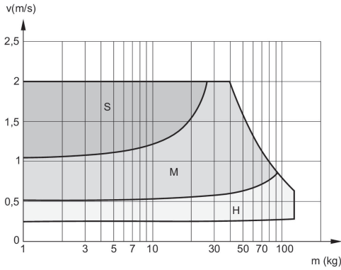
阻尼图 Ø 63 mm
