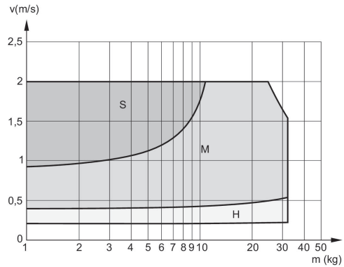
阻尼图 Ø 32 mm
