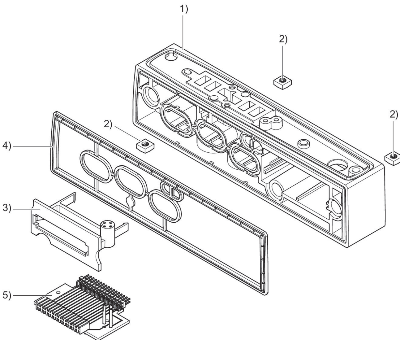
1) piastra di collegamento 2) tappi 3) supporto piastri 4) guarnizione sagomata 5) piastrina
