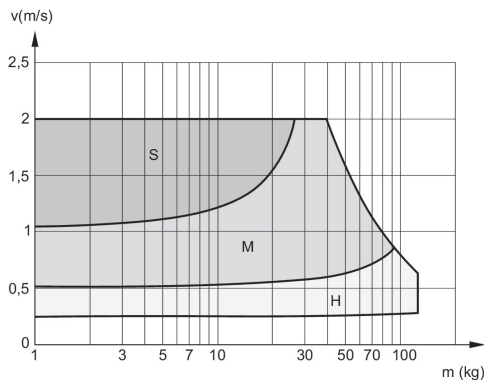
緩衝図表 Ø 63 mm
