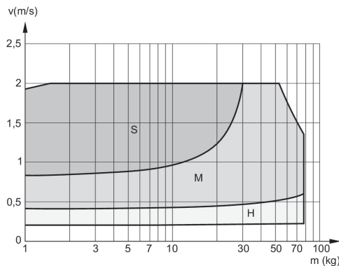
緩衝図表 Ø 50 mm
