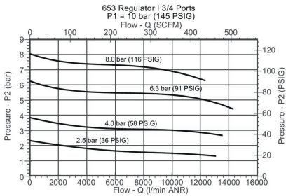
Diagramme du débit G 3/4
