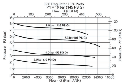
Diagrama de caudal G 3/4
