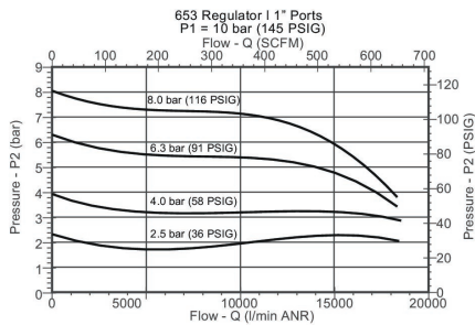
Diagrama de caudal G 1
